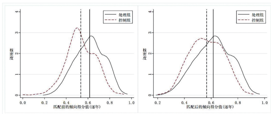
图2 匹配前后核密度曲线图
