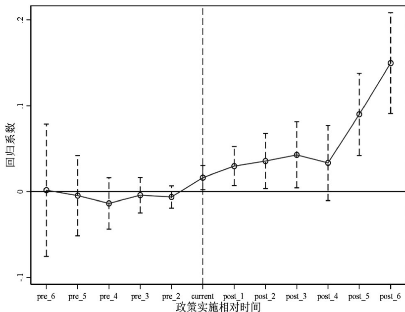
图3 平行趋势检验
