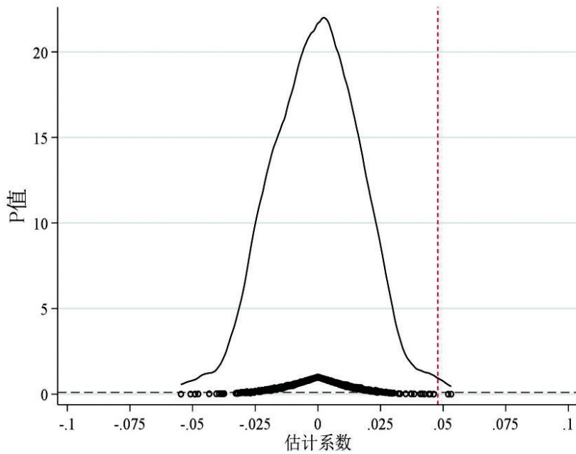
图4 安慰剂检验结果
